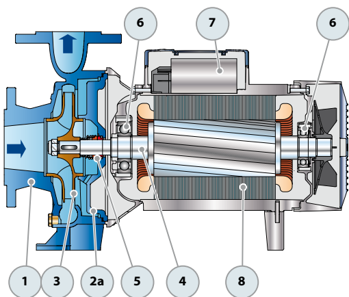
Versione monofase
