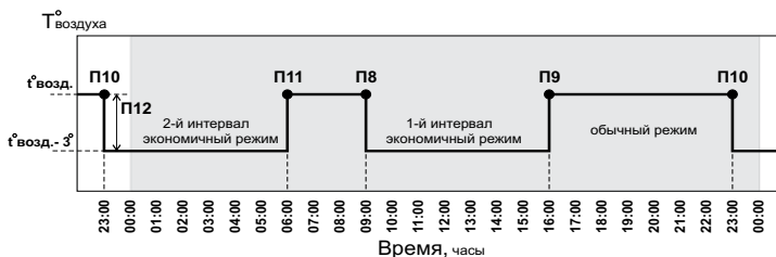
Рис.5 График температуры воздуха в помещении для Режимы 1.
