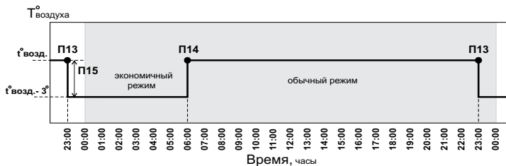
Рис.6 График температуры воздуха в помещении для Режимы 2.
