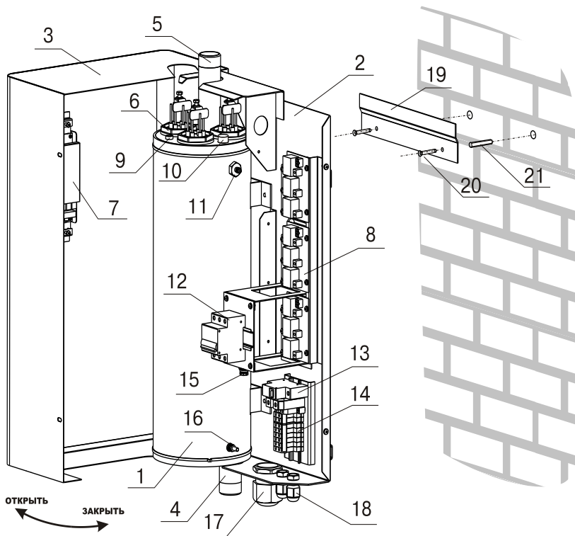
Рис.1 Конструкция электроводонагревателя и способ его крепления к стене
