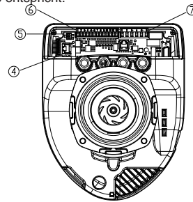
Abbildung 5: Elektroanschlüsse (Rückseite)
