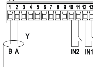
Obr. 7: Vyjímatelná 13 pólová svorkovnice: digitální vstupy a MODBUS
