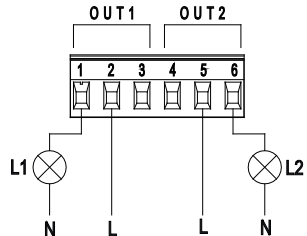
Obr. 9: Vyjímatelná 6 pólová svorkovnice: příklad připojení výstupů
