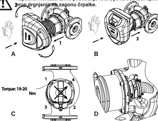
Slika 2: Navodilo za montažo glave motorja
