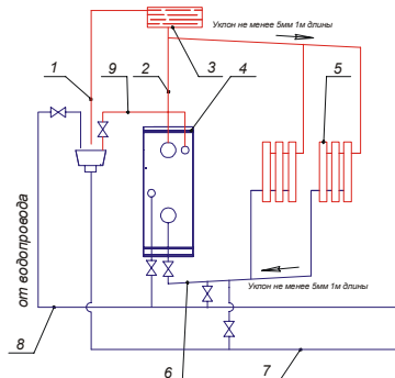
1 - сигнальная труба; 2 - главный стояк; 3 - расширительный бак; 4 - аппарат; 5 - радиатор; 6 - трубопровод обратной воды; 7 - сливная магистраль; 8 - подпиточный водопровод; 9 - трубопровод горячей воды;
