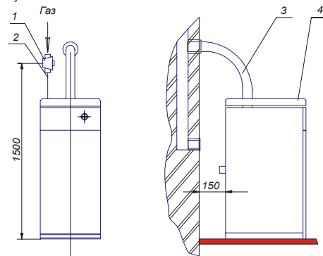
Рисунок 4 - Подключение аппарата к дымоходу и газопроводу
