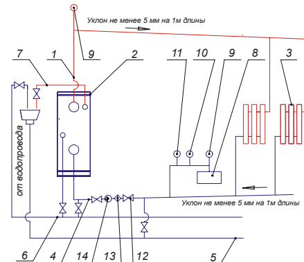
1 - главный стояк; 2- аппарат; 3- радиатор; 4- трубопровод обратной воды; 5- сливная магистраль; 6- подпиточный водопровод; 7- трубопровод горячей воды на бытовые нужды; 8- мембранный расширительный бак; 9- автоматический клапан выпуска воздуха; 10- манометр; 11- предохранительный клапан 150 кПа (1,5кас/см 2 ); 12- кран; 13- фильтр; 14- насос.
