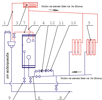
1 - сигнальная труба; 2 - главный стояк; 3 - расширительный бак; 4 - аппарат; 5 - радиатор; 6 - трубопровод обратной воды; 7-трубопровод горячей воды на бытовые нужды; 8 - сливная магистраль; 9 - подпиточный водопровод; 10- кран; 11- фильтр; 12- насос.
