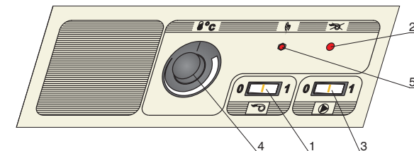
Рис.9. Панель пульта управления жидкотопливной/газовой горелкой (арт. 10230)
