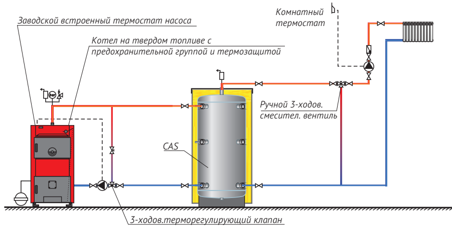
Рис.6. Пример установки котла ECO СК 70-110 кВт в закрытую систему отопления
