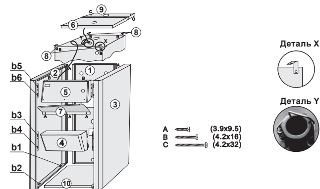
Рис.3. Порядок монтажа обшивки котла ECO CK 70-110 кВт
