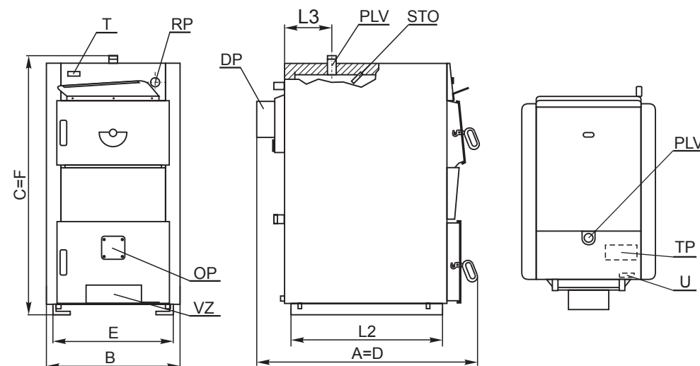
Рис.1. Вид котла ECO СК 70-110 кВт
