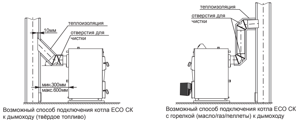
Рис.4. Возможный способ подключения котла ECO СК 70-110 кВт к дымоходу
