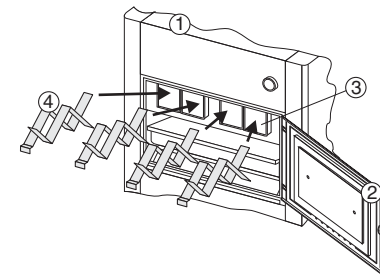
Рис.17. Установка турбулятора
