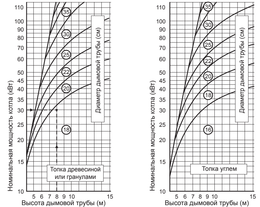
Рис.5. Размеры дымохода для котла ECO СК 70-110 кВт
