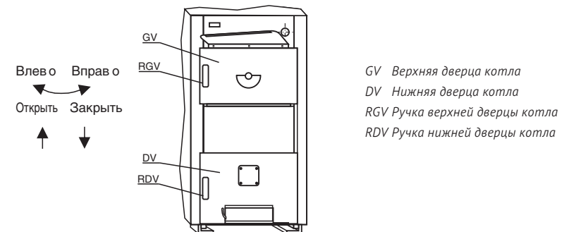
Рис.15. Процедура открытия дверей котла
