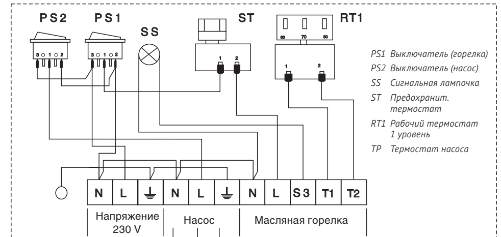
Рис.13. Электрическая схема регулировки котла ECO СК 70-110 кВт и термостата насоса при работе на жидком топливе /газе
