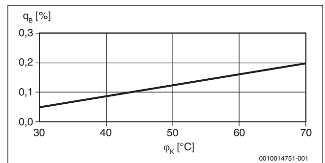
Рис. 45 Потери при эксплуатационной готовности в зависимости от средней температуры котла
