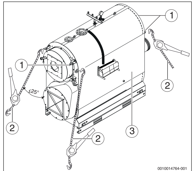
Рис. 3 Крепление котла при транспортировке
