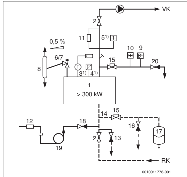
Рис. 43 Приборы безопасности по EN 12828:2012 для котлов мощностью > 300 кВт с предохранительным ограничителем температуры (STB) ≤ 110 °С
