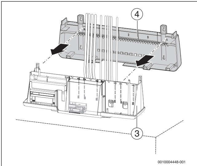
Рис. 32 Монтаж на котле, установка задней стенки
