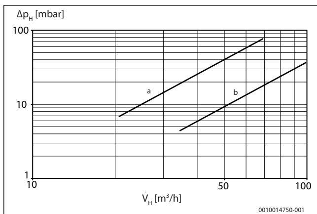
Рис. 44 Гидравлическое сопротивление водяного контура
