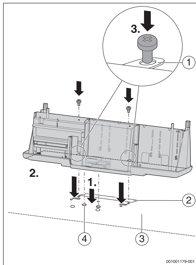
Рис. 29 Монтаж системы управления
