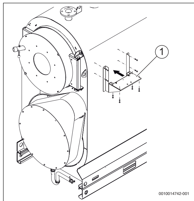
Рис. 30 Монтаж кронштейна системы управления
