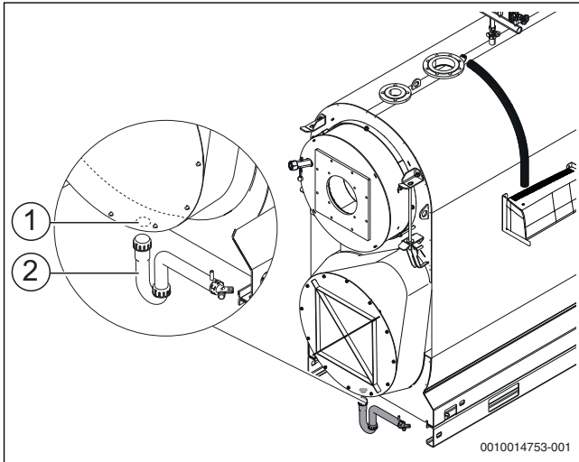
Рис. 41 Закрытие/открытие стока для чистящих средств
