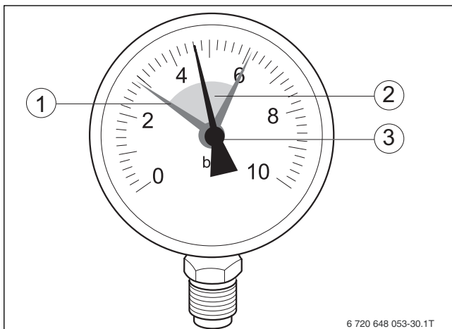
Рис. 42 Манометр для закрытых отопительных систем
