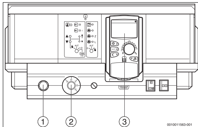
Рис. 28 Настройки системы управления
