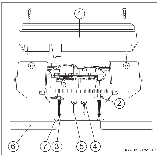
Рис. 24 Монтаж системы управления
