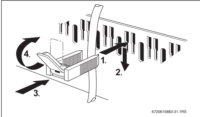
Рис. 31 Крепление провода хомутом
