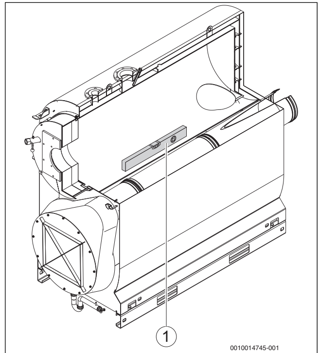
Рис. 11 Выравнивание котла
