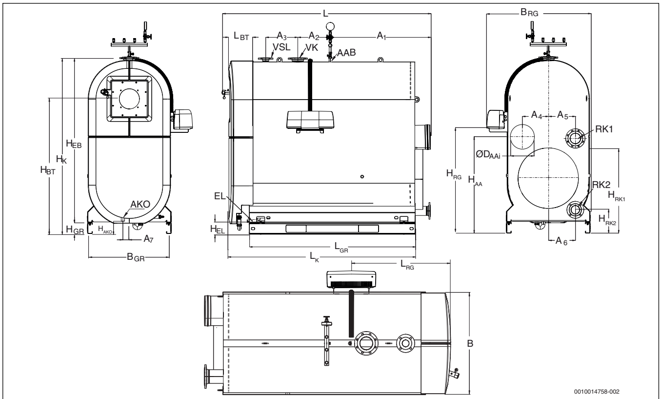
Рис. 2 Размеры и подключения
