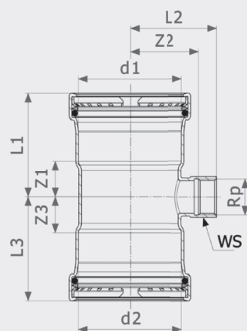
Тройник Sanpress Inox G XL - нержавеющая сталь Модель 0217.2XL
