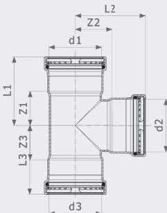
Тройник Sanpress Inox G XL - нержавеющая сталь Модель 0218XL
