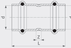
Муфта Sanpress Inox G - нержавеющая сталь Модель 0215
