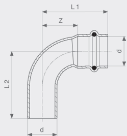
Отвод 90° Sanpress Inox G - нержавеющая сталь Модель 0216.1
