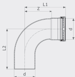
Отвод 90° Sanpress Inox G XL - нержавеющая сталь Модель 0216.1XL
