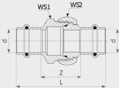
Соединительный элемент резьбовой Profipress G - бронза Модель 2650
