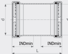
Надвижная муфта Sanpress Inox G XL - нержавеющая сталь Модель 0215.5XL
