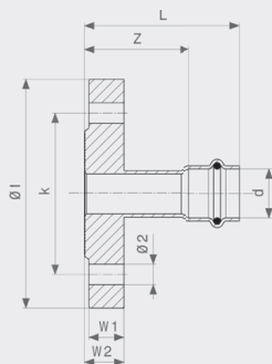
Фланцевый переход Sanpress Inox G - нержавеющая сталь Модель 0259
