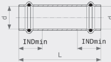
Надвижная муфта Sanpress Inox G - нержавеющая сталь Модель 0215.5
