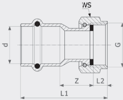
Переход на резьбовые соединения Profipress G - бронза Модель 2666
