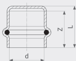
Заглушка Sanpress Inox G - нержавеющая сталь Модель 0256
