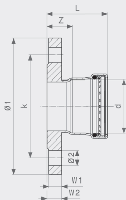
Фланцевый переход Sanpress Inox G XL - нержавеющая сталь Модель 0259XL
