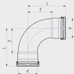
Отвод 90° Sanpress Inox G XL - нержавеющая сталь Модель 0216XL
