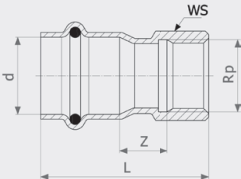
Соединительный элемент Sanpress Inox G - нержавеющая сталь Модель 0212
