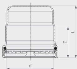
Заглушка Sanpress Inox G XL - нержавеющая сталь Модель 0256.1XL
