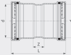
Муфта Sanpress Inox G XL - нержавеющая сталь Модель 0215XL
