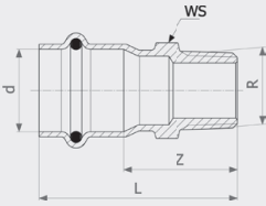
Соединительный элемент Sanpress Inox G - нержавеющая сталь Модель 0211
