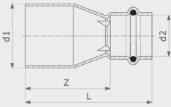
Редукционная вставка Sanpress Inox G - нержавеющая сталь Модель 0215.1
