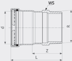
Соединительный элемент Sanpress Inox G XL - нержавеющая сталь Модель 0211XL
