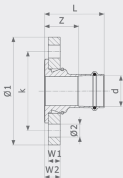
Фланцевый переход Profipress G - бронза Модель 2659.5
