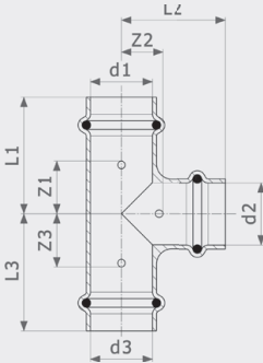
Тройник Sanpress Inox G - нержавеющая сталь Модель 0218
