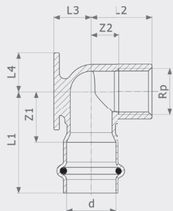
Водорозетка Sanpress Inox G - нержавеющая сталь Модель 0225.5
