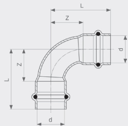
Отвод 90° Sanpress Inox G - нержавеющая сталь Модель 0216
