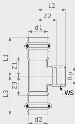
Тройник Sanpress Inox G - нержавеющая сталь Модель 0217.2
