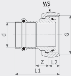
Переход на резьбовые соединения Profipress G - бронза Модель 2661
