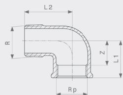
Присоединительный угольник 90° - бронза Модель 2614.5
