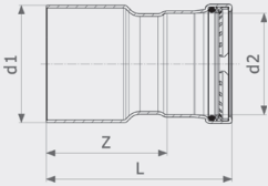
Редукционная вставка Sanpress Inox G XL - нержавеющая сталь Модель 0215.1XL
