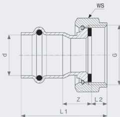
Переход на резьбовые соединения Sanpress Inox G - нержавеющая сталь Модель 0263.1
