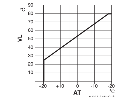
Рис 12 Основная настройка отопительной кривой для метода начальной/конечной точек
