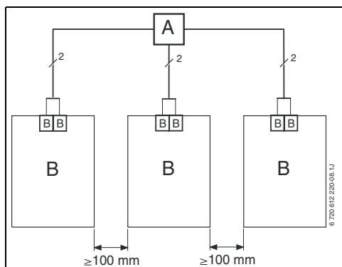
Рис 10 Подсоединение соединений с BUS-шиной через ответвительную коробку (A)
