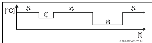
Рис 11 Пример программы горячая вода с профилем времени и уровня температуры
