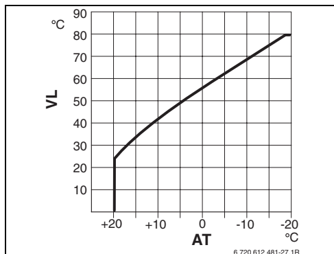
Рис 14 Основная настройка отопительной кривой для подогрева с использованием радиаторов
