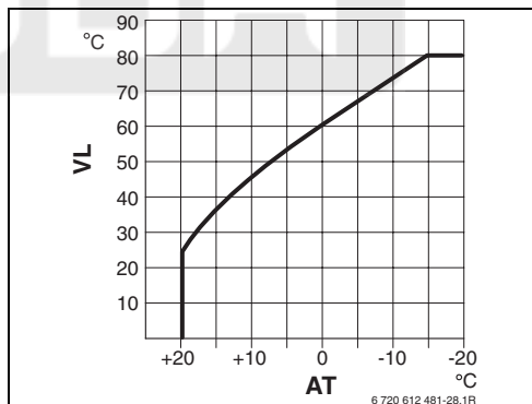
Рис 15 Основная настройка отопительной кривой для подогрева с использованием конвекторов
