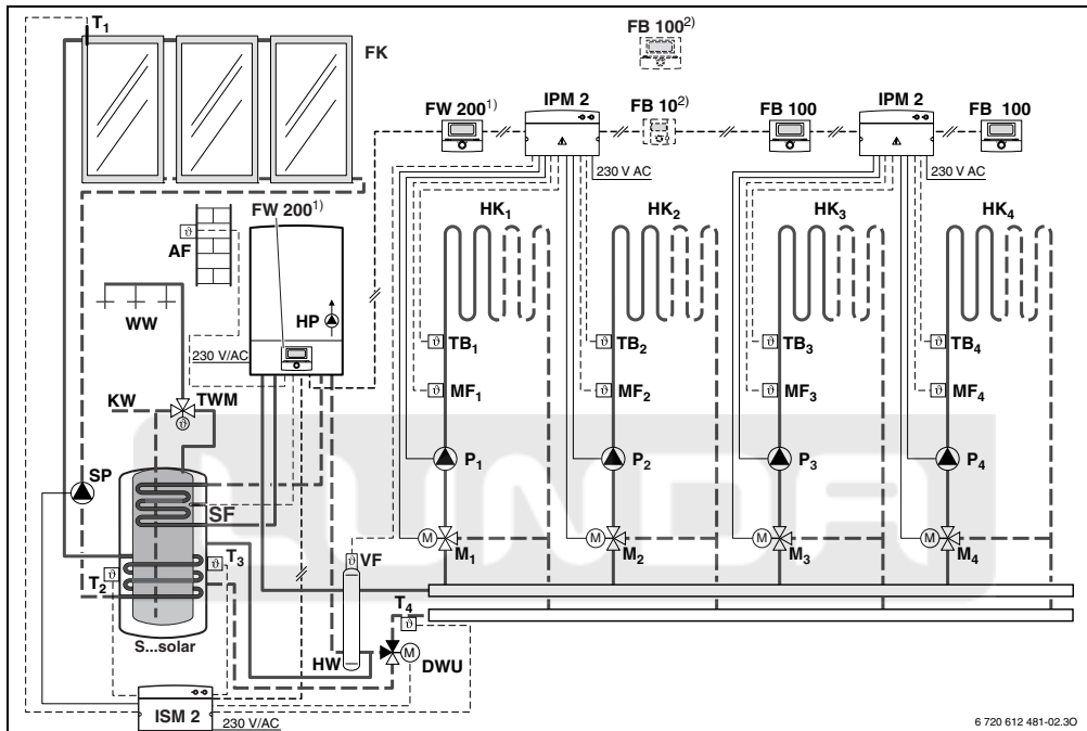
Рис 4 Упрощённая схема установки (схема, предусмотренная для монтажа и прочие возможности в плановой документации)
