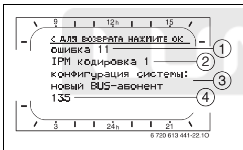
Рис 16 Индикация ошибки
