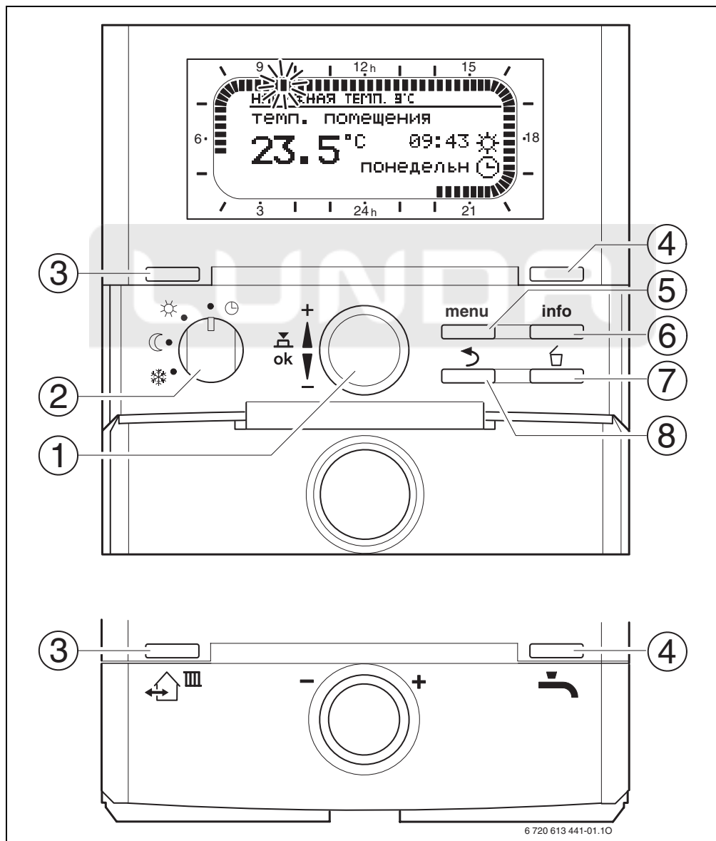
Рис 1 Стандартный дисплей
