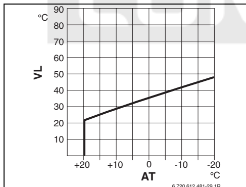
Рис 13 Основная настройка отопительной кривой для обогрева пола
