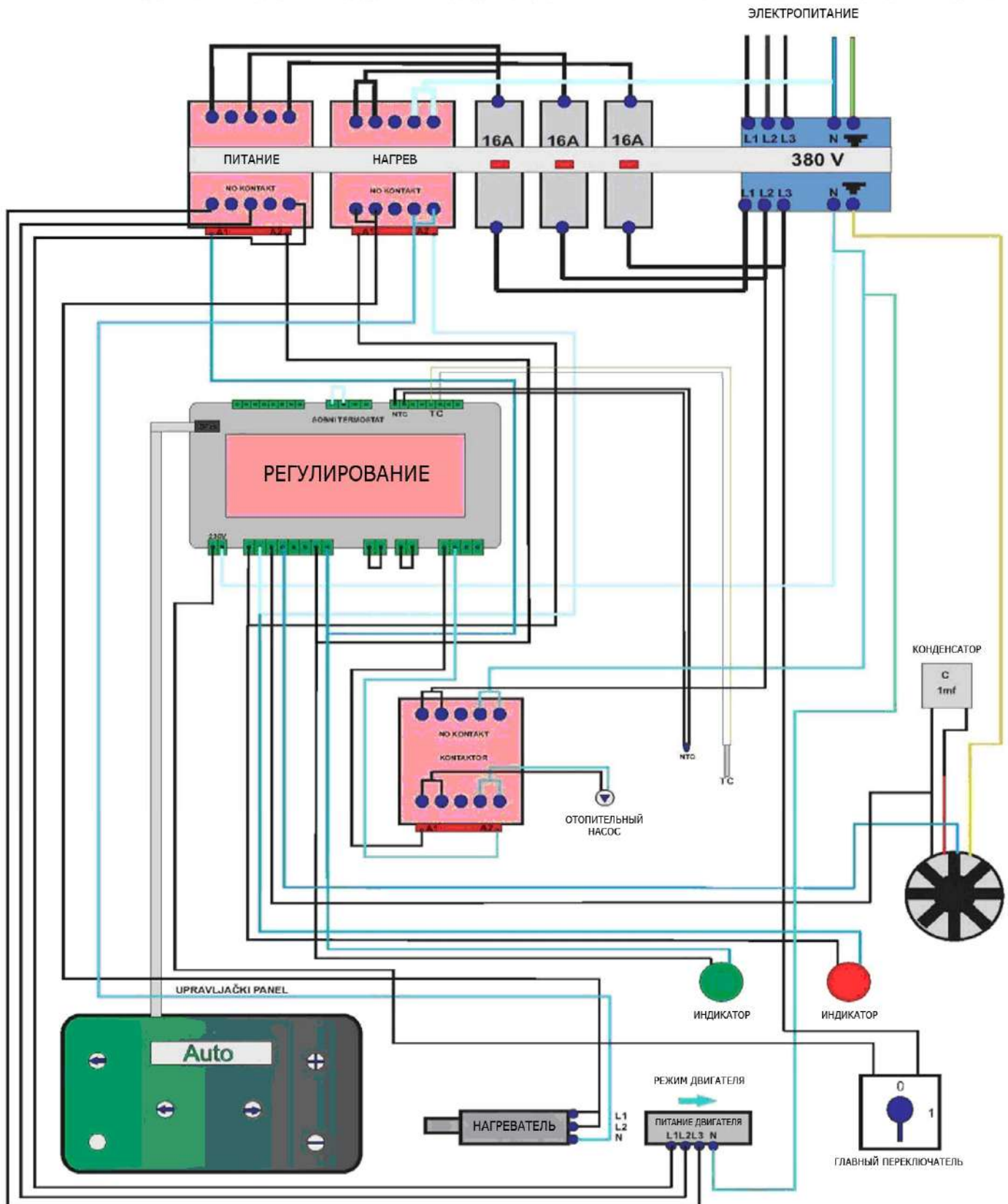
Рисунок 18: Электрическая схема
