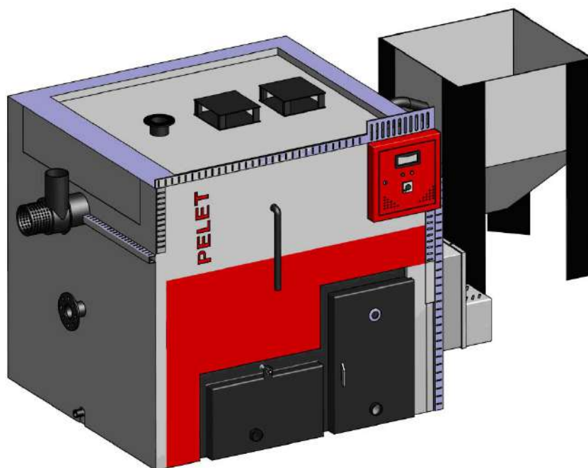
Рисунок 1. Вид котла WIRBEL™ ECO SMK 150÷300 кВт в аксонометрии (с бункером)
