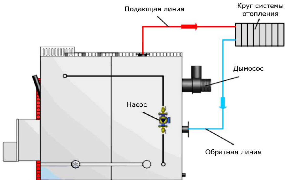
Рисунок 8. Гидравлическая схема подключения
