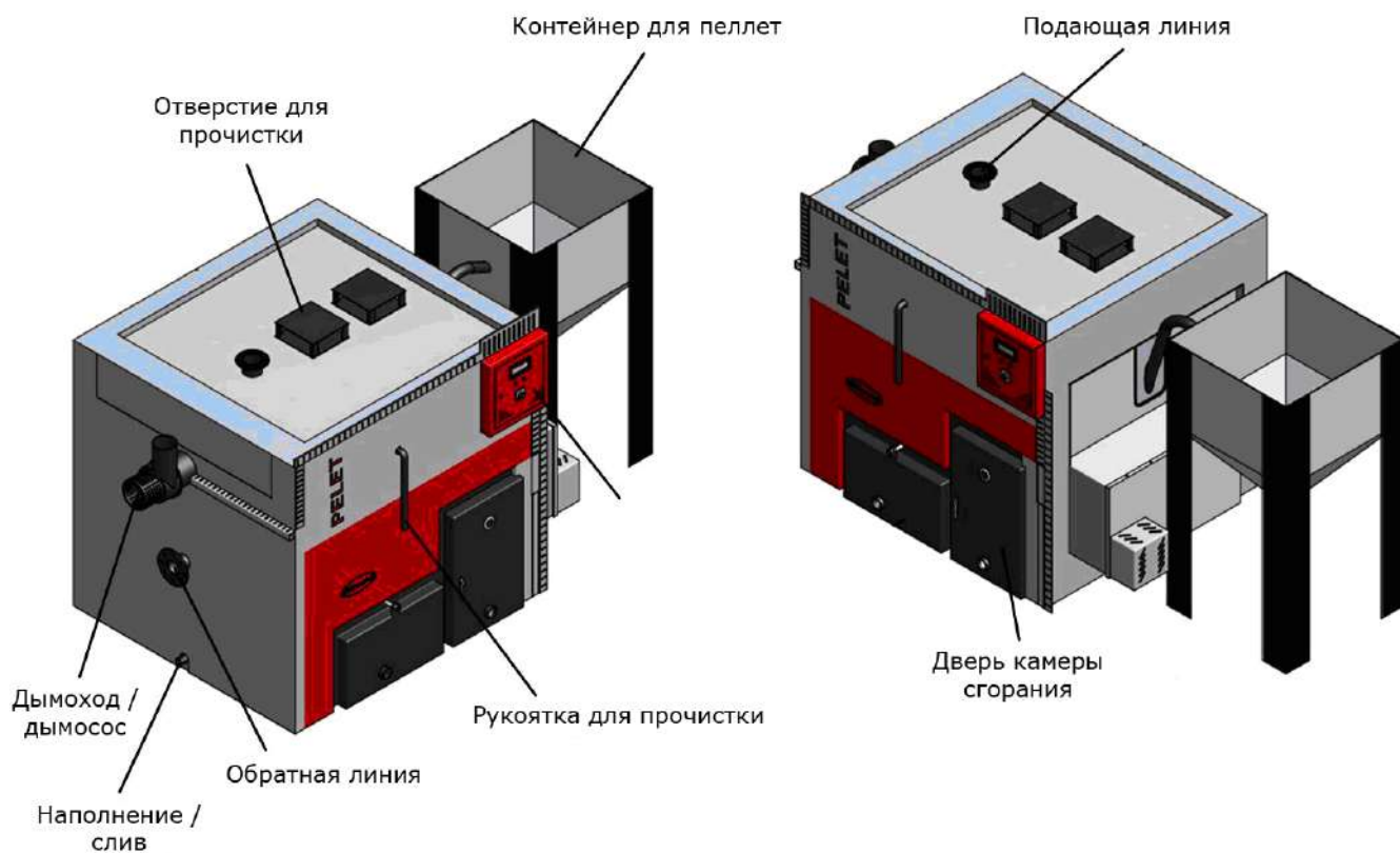
Рисунок 4. Основные части котла WIRBEL™ ECO SMK 150÷300 кВт
