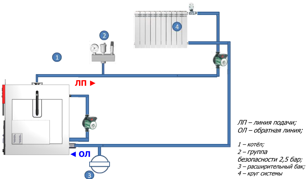
Рисунок 9. Гидравлическая схема подключения
