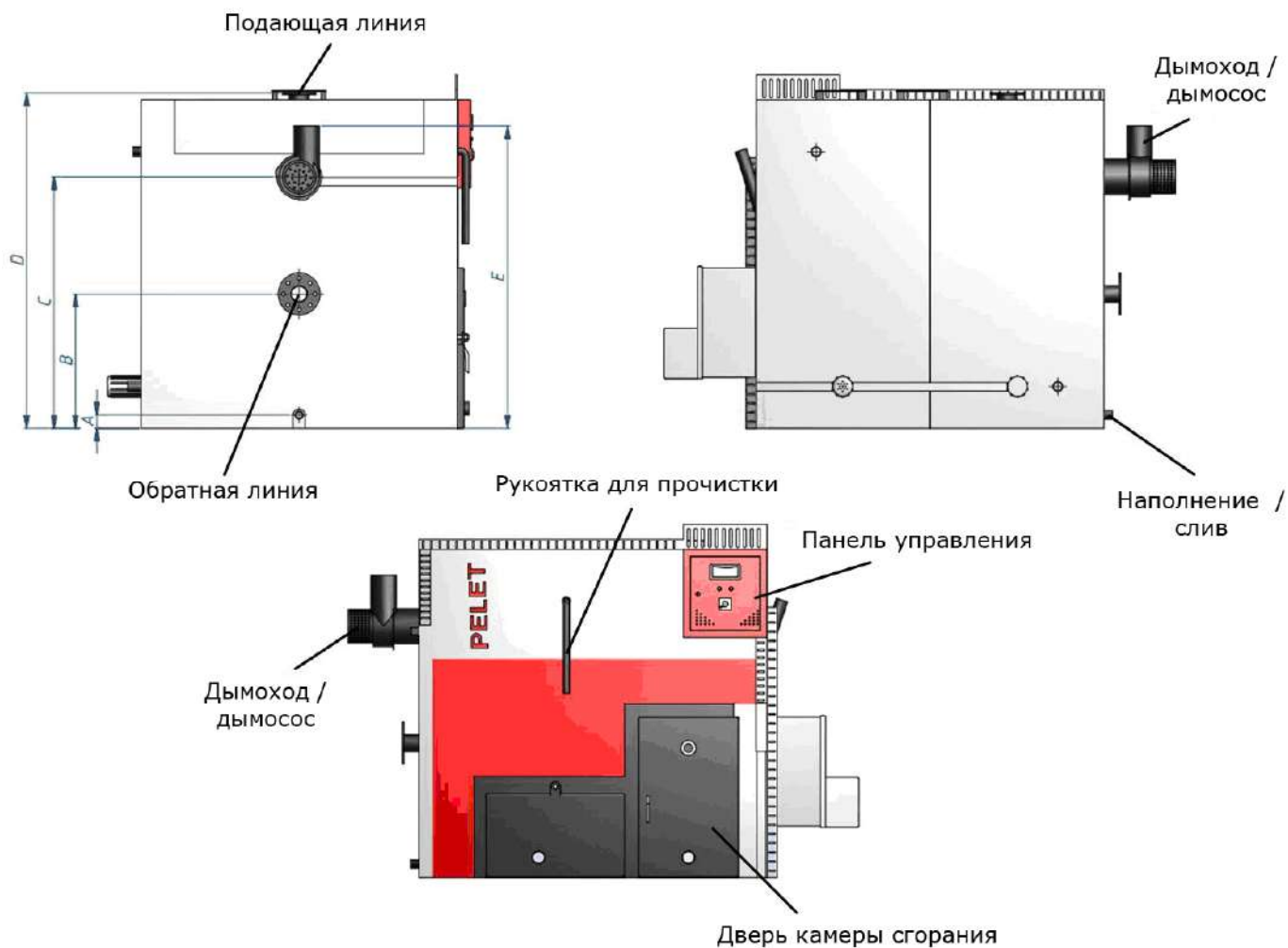
Рисунок 3. Вид и размеры котла WIRBEL™ ECO SMK 150÷300 кВт
