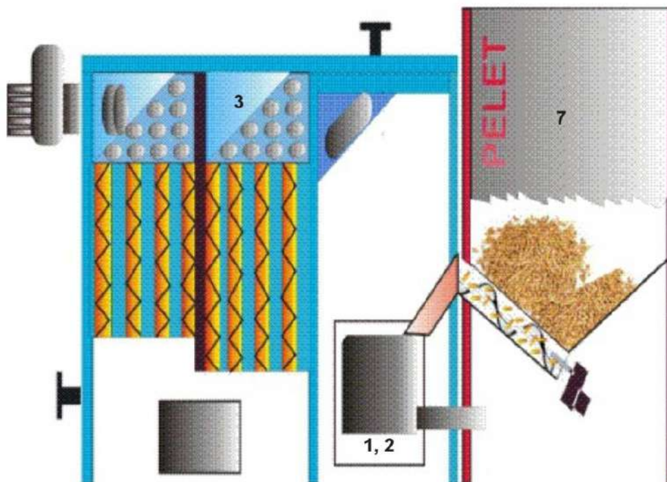
Рисунок 5. Поперечное сечение котла WIRBEL™ ECO SMK 150÷300 кВт
