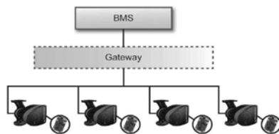
46-сур. Параллель қосылған төрт сорғылы үй ішілік коммуникацияларды басқару жүйесі (BMS)
