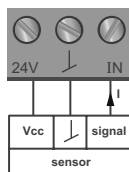
26-сур. Сыртқы датчикке арналған ұқсас кіріс, 4-20 мА сигналы
