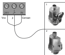
27-сур. Сыртқы датчиктер мысалдары
