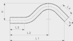
Одноплоскостной обводной элемент Sanpress - нержавеющая сталь Модель 2209.3
