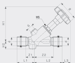
Наклонный вентиль Easytop Inox - нержавеющая сталь Модель 2337
