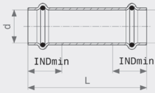
Надвигная муфта Sanpress Inox - нержавеющая сталь Модель 2315.5
