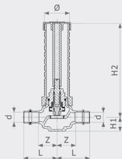
Вентиль скрытого монтажа Easypot Модель 2235
