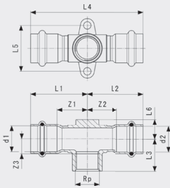
Тройник-водорозетка Sanpress Inox - нержавеющая сталь Модель 2317.3
