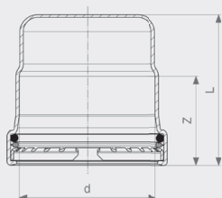
Заглушка Sanpress Inox XL - нержавеющая сталь Модель 2356.1XL
