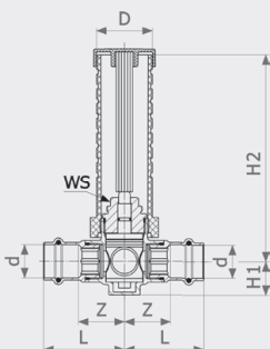
Шаровый кран полнопроходной для скрытого монтажа Easytop Модель 2240
