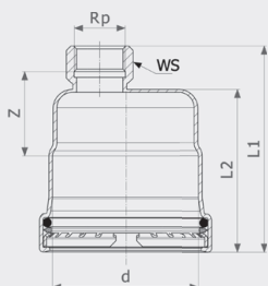
Заглушка Sanpress Inox XL - нержавеющая сталь Модель 2356XL
