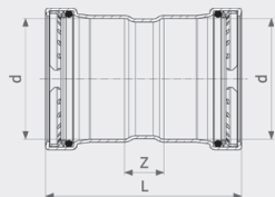
Муфта Sanpress Inox XL - нержавеющая сталь Модель 2315XL
