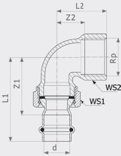
Переходной элемент 90° Sanpress Inox - нержавеющая сталь Модель 2355
