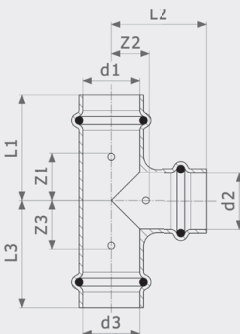
Тройник Sanpress Inox - нержавеющая сталь Модель 2318
