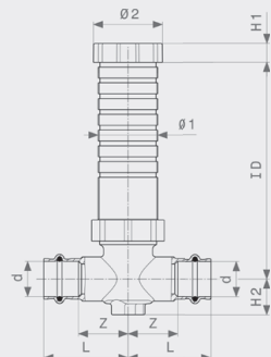
Шаровой кран полнопроходной для скрытого монтажа Easypot Модель 2278.5
