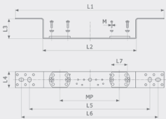
Монтажная консоль - сталь оцинкованная Модель 2021.7
