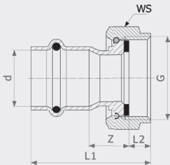
Переход на резьбовые соединения Sanpress Inox - нержавеющая сталь Модель 2363
