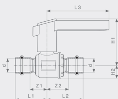
Шаровый кран Easytop Inox Модель 2370
