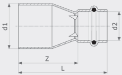
Редукционная вставка Sanpress Inox - нержавеющая сталь Модель 2315.1
