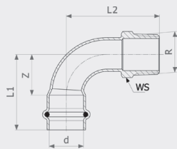
Угольник переходной 90° Sanpress Inox - нержавеющая сталь Модель 2314
