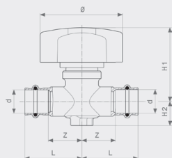
Шаровый кран полнопроходной Easytop Модель 2278
