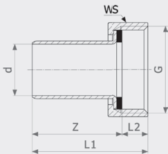
Переход на резьбовые соединения Sanpress Inox - нержавеющая сталь Модель 2364
