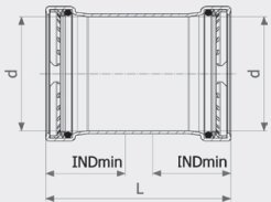
Надвигная муфта Sanpress Inox XL - нержавеющая сталь Модель 2315.5XL
