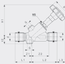
CRV наклонный вентиль свободного потока Easytop Inox - нержавеющая сталь Модель 2338
