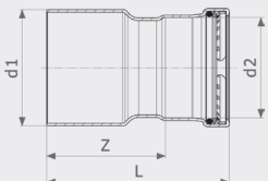
Редукционная вставка Sanpress Inox XL - нержавеющая сталь Модель 2315.1XL
