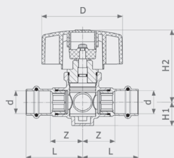
Шаровый кран полнопроходной Easytop Модель 2242
