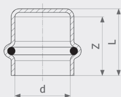
Заглушка Sanpress Inox - нержавеющая сталь Модель 2356
