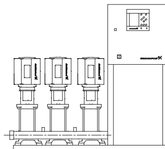
25-сур. Кіріктірілген ИП-реттеуішпен (тұйықталған контур) реттелетін қондырғы.
