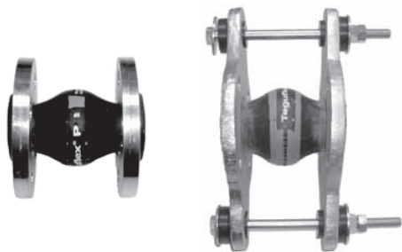
8-сур. Резеңке аралық қабаттармен шектеуші тұтастырғыштарсыз және олармен діріл ендірімелері
