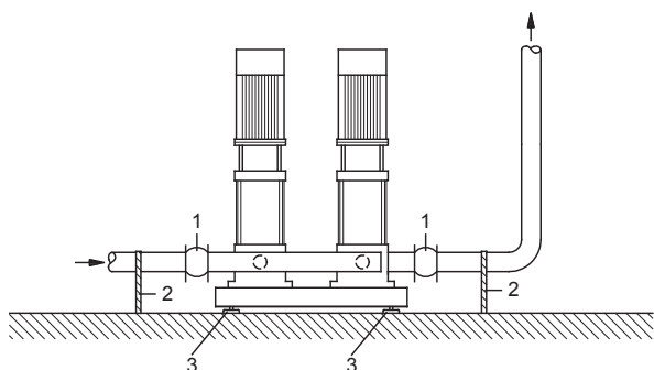
6-сур. Титирөөгө койгучтардын, түтүктөр үчүн тирөөчтөрдүн жана титирөө тирөөчтөрүнүн абалы
