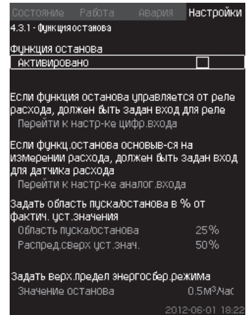
Рис. 69 Функция останова
