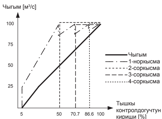
30-сур. MPC-F үчүн ачык чөйрөсүзүк үчүн жөнгө салуучу мүнөздөмө
