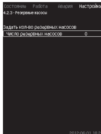
60-сур. Камдык соркысмалар
