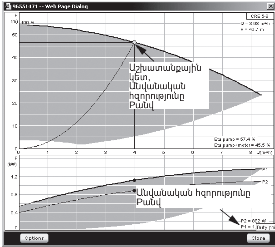
Նկար 96 Անվանական հզորության ցուցմունքը P_{անվանական} Q_{անվանական} և H_{անվանական} - պոմպերի անվանական աշխատանքային կետ և, որպես օրենք, դա ամենաբարձր ՕԳԳ-ով կետն է:
