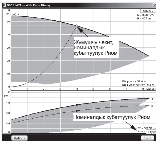
96-сур. Показание номиналдык кубаттуулуктун P_{ном} көрсөткүчү Q_{ном} жана H_{ном} – соркысмалардын номиналдык жумушчу чекити жана эреже катары бул эң жогорку ПАК менен жумушчу чекит.
