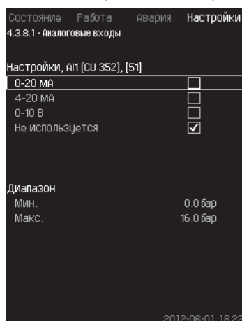
Рис. 81 Аналоговые входы
