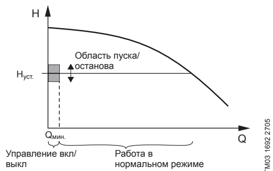
Рис. 70 Область пуска/останова
