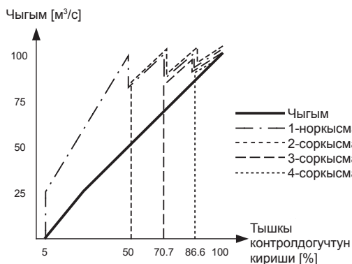
28-сур. Ачык чөйрөсүзүк үчүн жөнгө салуучу мүнөздөмө
