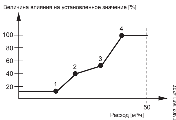
Рис. 47 Соотношение между влиянием на установленное значение и расходом
