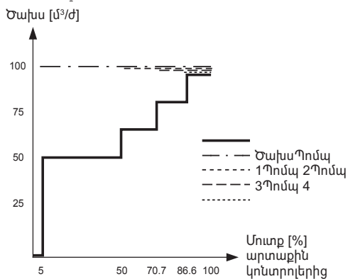
Նկար 30 Կարգավորման բնութագիր MPC-F-ի համար անջատված կոնտուրում
