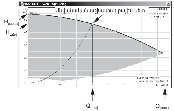
Նկար 93 Ցուցումներ Q_{անվանական} , H_{անվանական} , H_{առավելագույն} և Q_{առավելագույն}
