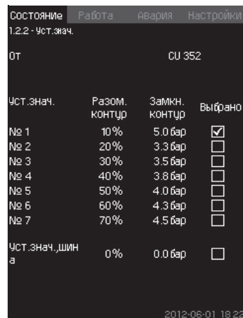
Рис. 15 Устан. значение
