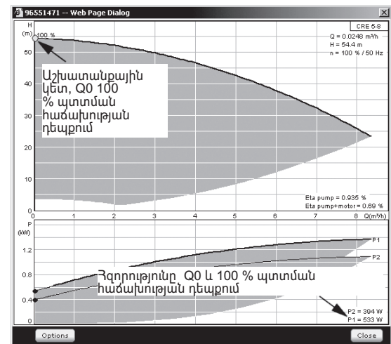
Նկար 93 Ցուցումներ Q_{անվանական} , H_{անվանական} , H_{առավելագույն} և Q_{առավելագույն}
