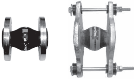
8-сур. Чектөөчү тарткычтарсыз жана алар менен резина төшөмөлүү титирөөгө койгучтар
