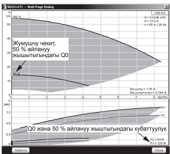
95-сур. Кубаттуулуктун Q0 жана 50 % айлануу жыштыгындагы көрсөткүчү
