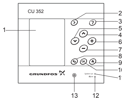
Рис. 9 Панель управления
