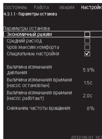
Рис. 73 Специальные настройки
