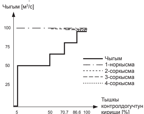
31-сур. MPC-S үчүн ачык чөйрөсүзүк үчүн жөнгө салуучу мүнөздөмө
