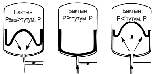
5-сүр. Мембраналык оргутуучу бак (P-басым)
