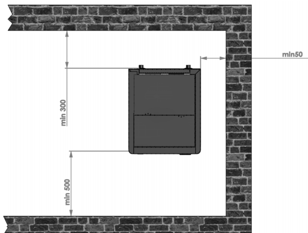
Рисунок 3. Расположение котла в помещении
