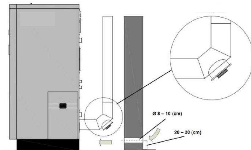
Рисунок 2. Минимальные промежутки для установки вентиляционных решёток
