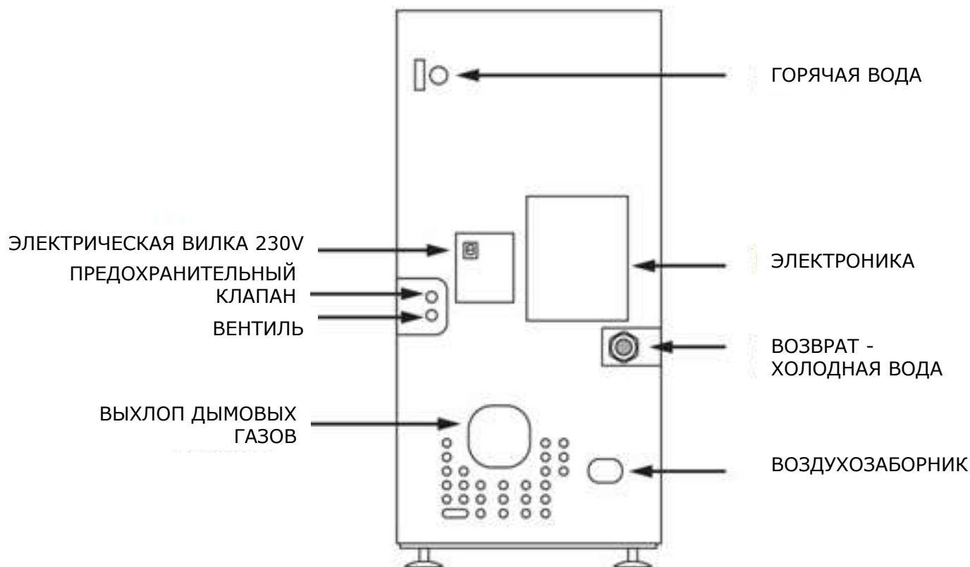
Рисунок 10. Задняя часть котла с разъемами
