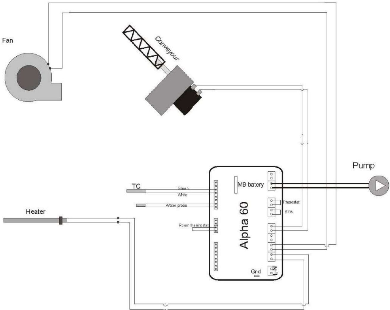
Рисунок 30: Электрическая схема
