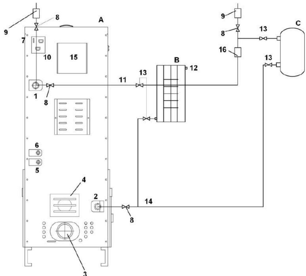
Рисунок 9. Гидравлическая схема подключения
